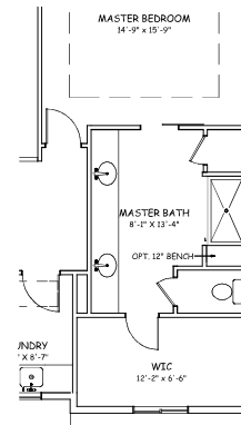
OPTIONAL MASTER BATH
