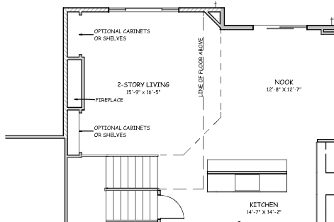
OPTIONAL FIREPLACE 2 LAYOUT
